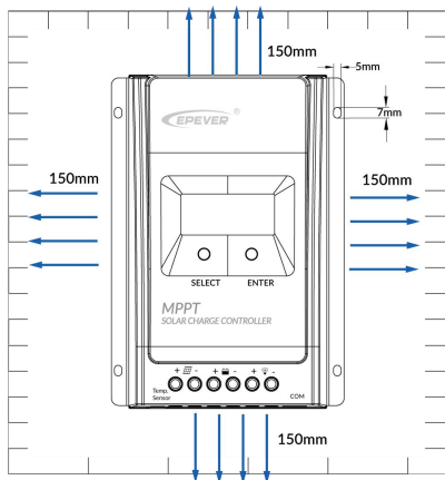
图2-1安装示意图
